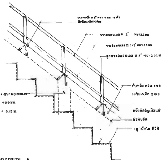
แบบขยาย 3 ขนาดจริง 1:10
