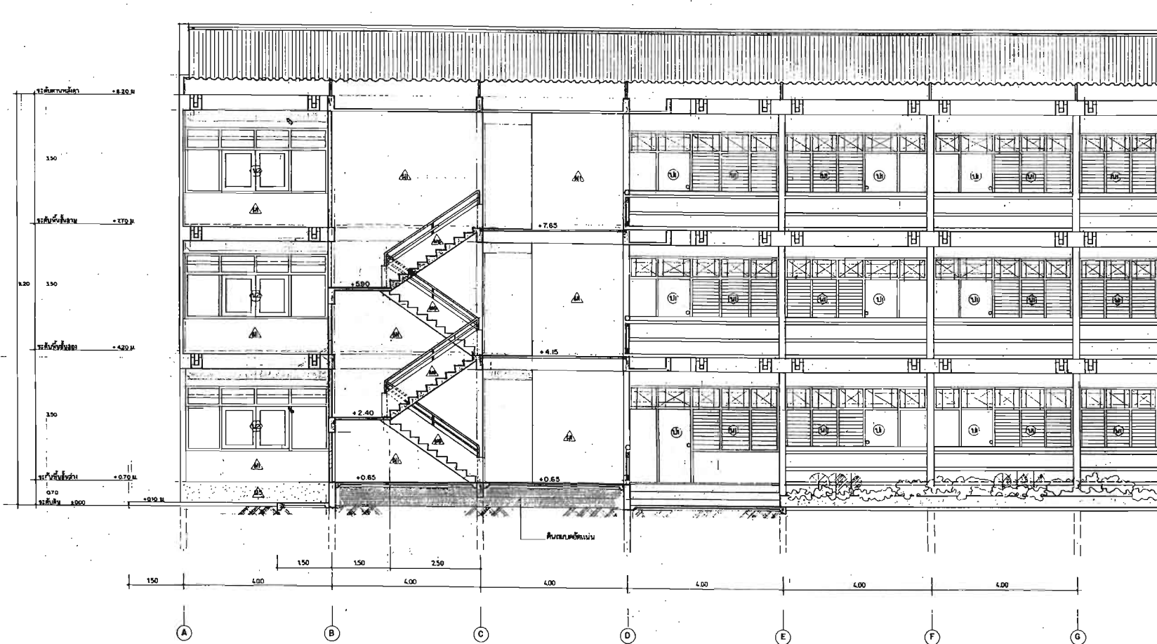
รูปตัดตามแนว (A) - (B) มาตราส่วน 1:150
