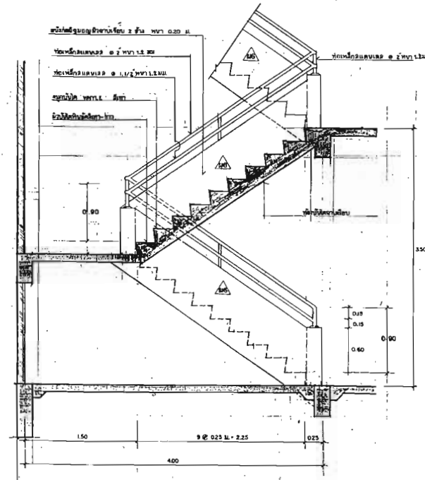
รูปตัด (1-1) มาตราส่วน 1:25
