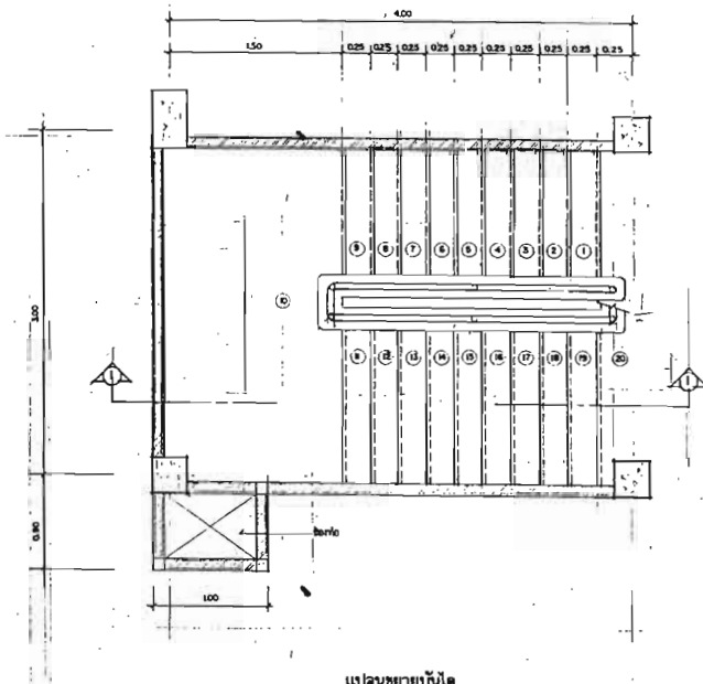
แปลนขยายบันได มาตราส่วน 1:25
