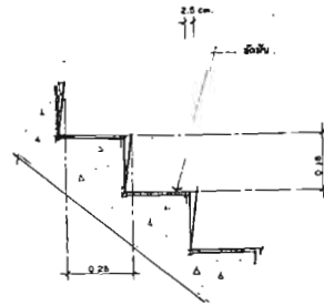
แบบขยาย ขนาดจริง 1:10
