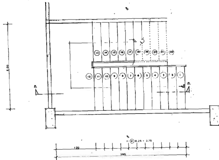
แบบขยายบันได 1 ขนาดจริง 1:25
