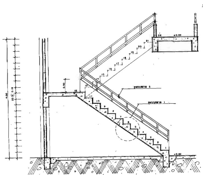
รูปตัด ก-ก ขนาดจริง 1:25
