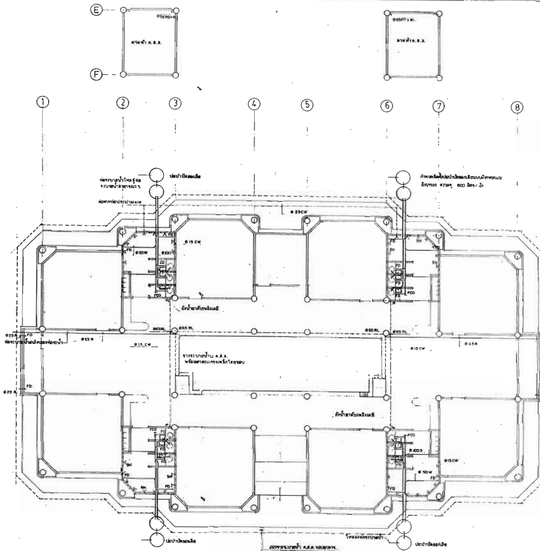
ผังประปาพื้นชั้นล่าง มาตราส่วน 1:100
