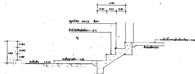
ขยายบันไดทางขึ้นหน้าอาคาร มาตราส่วน 1:25
